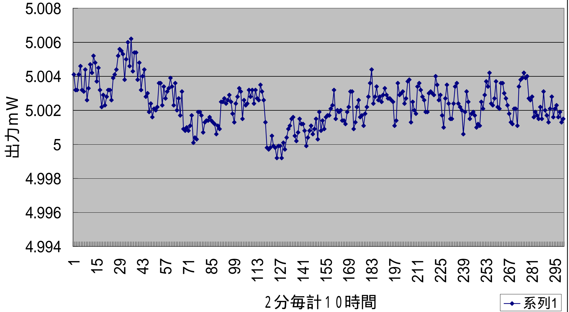
10時間試験 (センサQ82321) 650nm5mW-APC駆動 コア4 \mu mSMF接続
