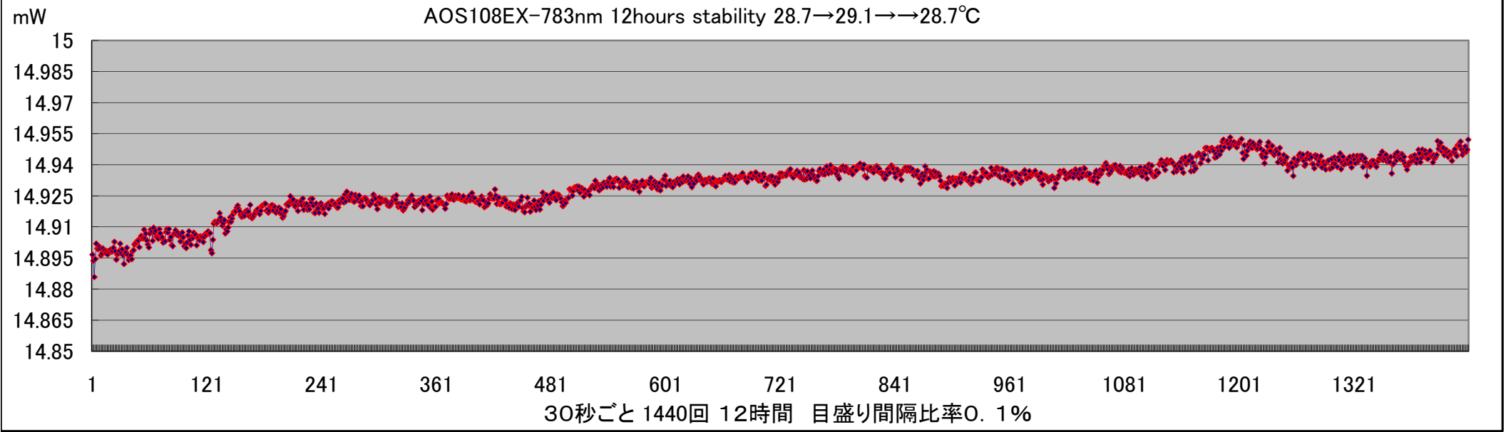
AOS108-783nmEX経時変化データ(温調無し、エアコンOFFの状態)
